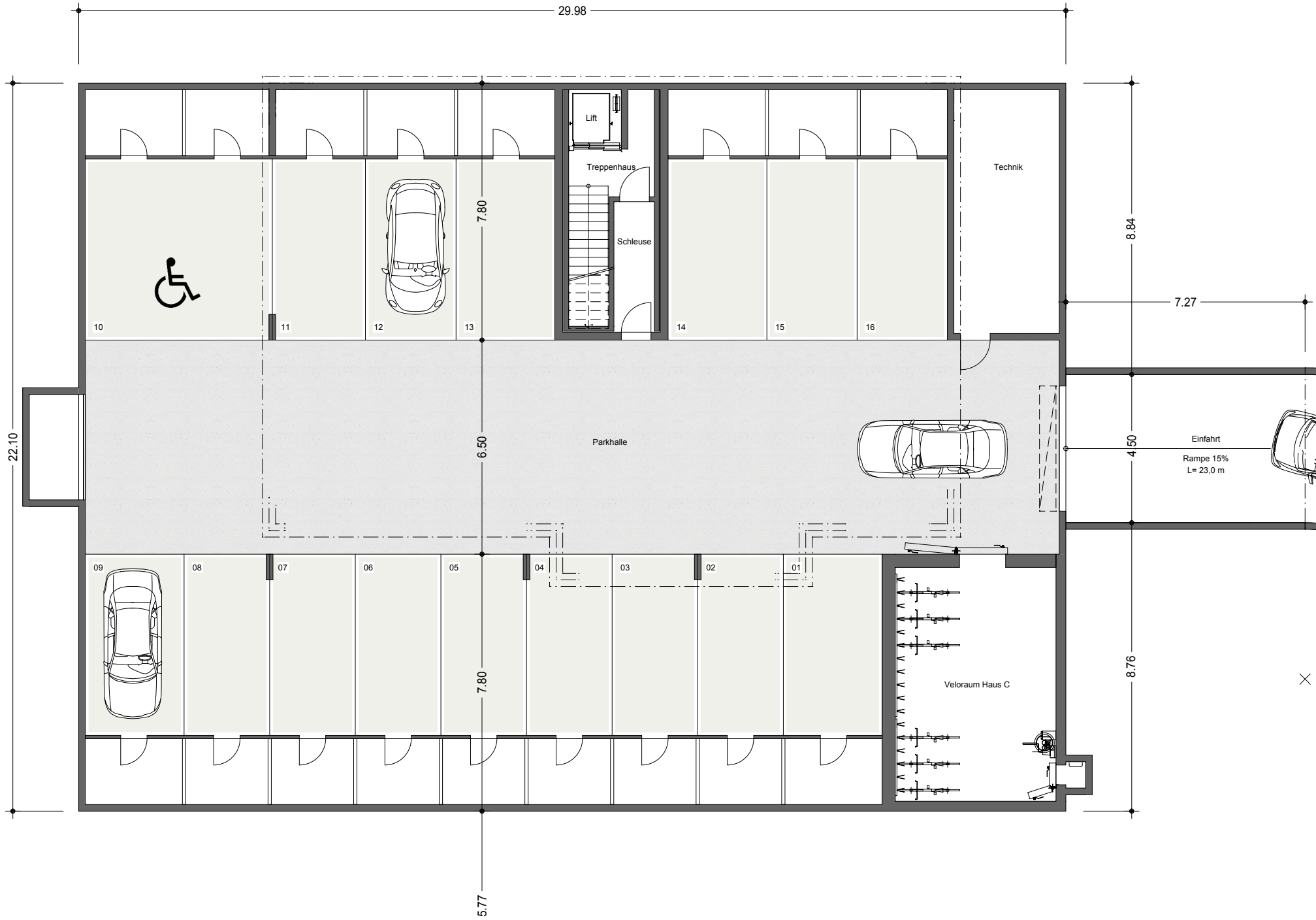
Untergeschoss Haus C 1:150
